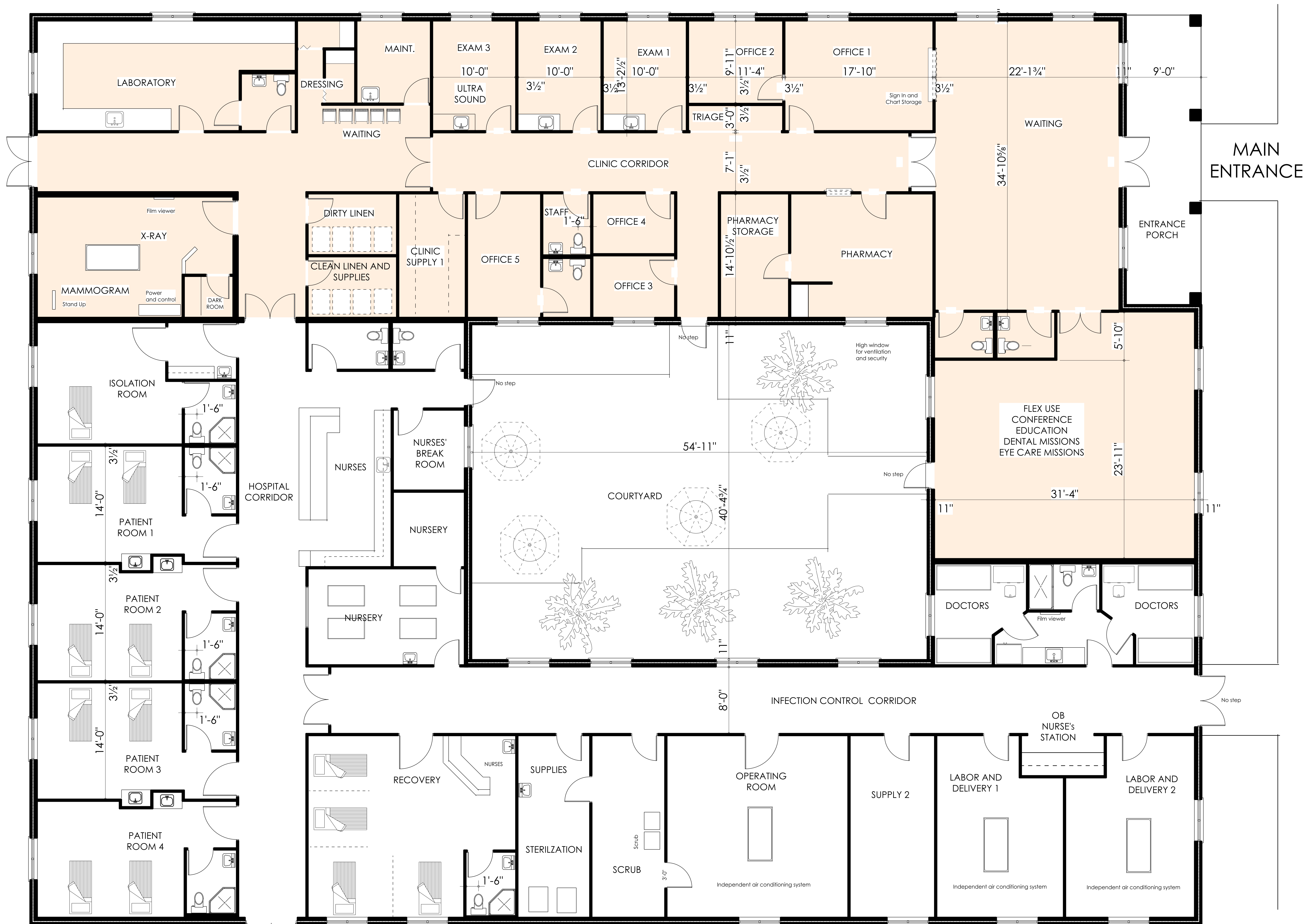
FLOOR PLAN PLANTA BAJA
